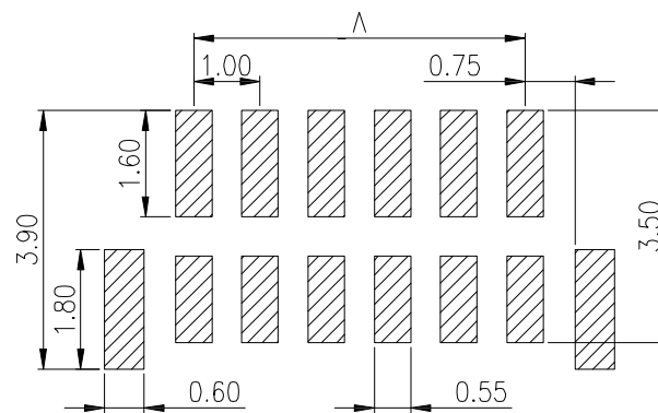
P.C.B Layout
