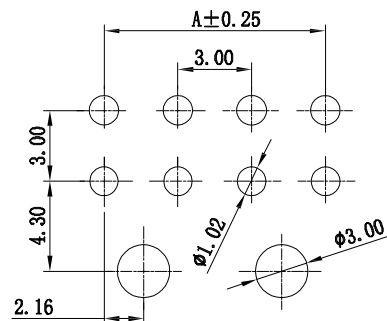
8P~24P P.C.B LAYOUT
