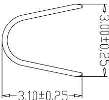
SEC:A-A
