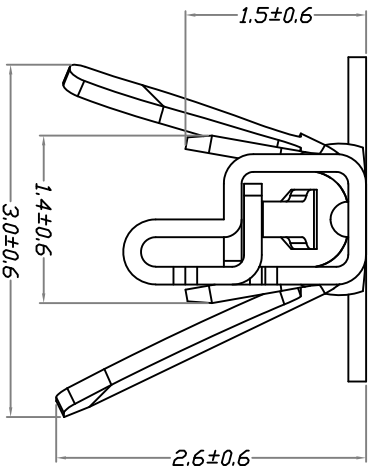
A处放大图 4:1
